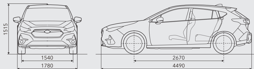
Dimensions selon normes de mesure de SUBARU CORPORATION.
